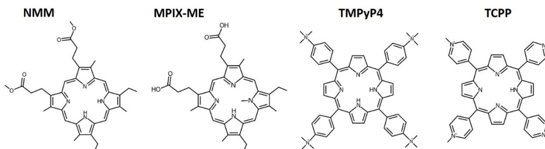
Obrázek 1. Struktury porfyrinů používaných v tomto funkčním vzorku.
