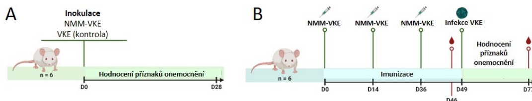
Obrázek 2. Schémata in vivo experimentů. (A) Test virulence VKE inaktivovaného porfyrinem NMM v myším modelu. VKE ošetřený porfyrinem NMM a kontrolní VKE (ošetřený PBS) byl injikován myším kmene BALB/c, klinická skóre a mortalita byly monitorovány až do 28. dne po infekci. (B) Ověření ochranného účinku VKE inaktivovaného porfyrinem NMM u myši. VKE inaktivovaný porfyrinem NMM byl použit k imunizaci myši kmene BALB/c. Myši byly následně vystaveny letální infekční dávce VKE, přičemž bylo sledováno klinické skóre a mortalita. Ve stanovených dnech byly odebrány vzorky krve a stanovováno množství protilátek proti VKE (symboly červených kapek) (upraveno dle Holoubek et al., 2024).
