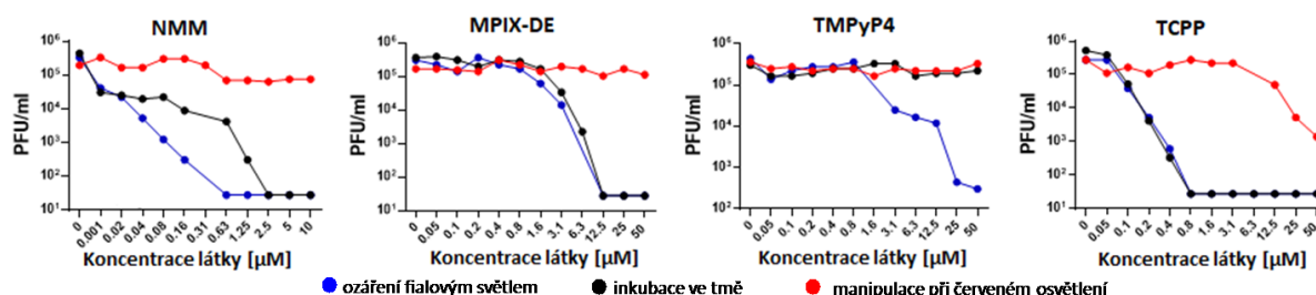
Obrázek 6. Světlem indukovaná virus-inaktivační aktivita vybraných porfyrinů. U NMM byla zjištěna EC_{50} při inkubaci ve tmě 0.173 \mu\text{M} (černá křivka), zatímco po ozáření fialovým světlem 0.049 \mu\text{M} (modrá křivka, vzrůst aktivity 3.5krát). Pro srovnání u TCPP byly zjištěny EC_{50} ve tmě 0.202 \mu\text{M} (černá křivka) a po ozáření 0.233 \mu\text{M} (modrá křivka, tj. téměř žádný rozdíl v aktivitě) (upraveno dle Holoubek et al., 2024).
